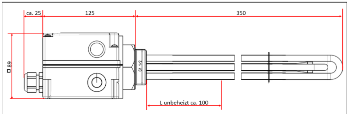
Abbildung 7: Abmessungen Einschraubheizkörper für PV und Netzbetrieb
